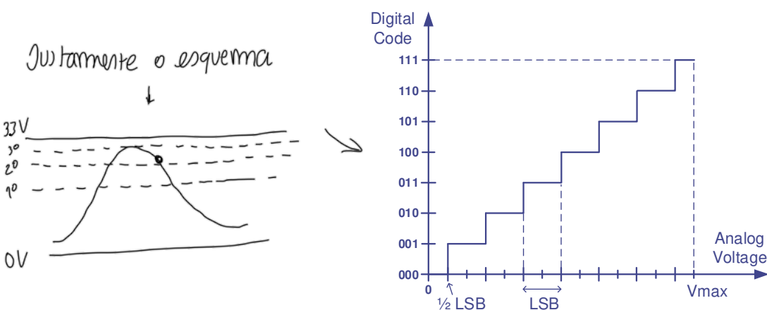
Figura 1. Conversão de uma gama de tensão 0 - V_{max} com 3 bits (8 níveis).
